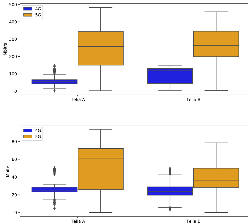
Figur 5.2: Nedlastingshastighet (øverst) og opplastingshastighet (nederst) for 5G målenoder i Telias nett.
