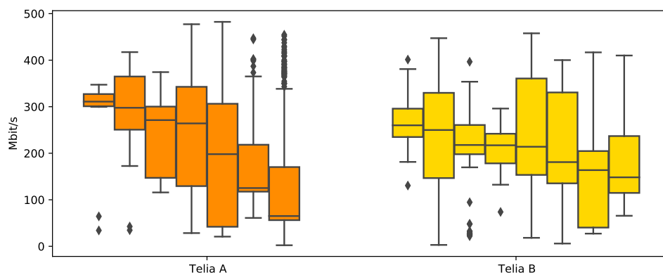
Figur 5.3: Nedlastingshastighet i forskjellige celler for 5G målenoder i Telias nett.
