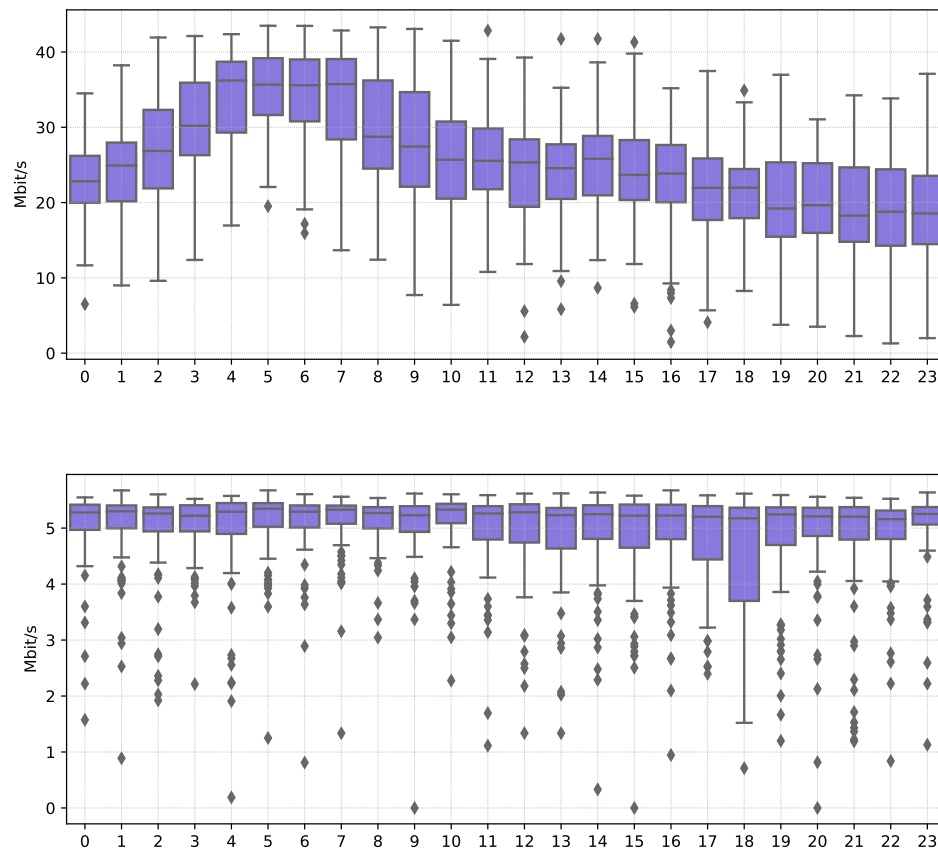
Figur 6.3: Nedlastingshastighet (øverst) og opplastingshastighet (nederst) over satellittforbindelse.
