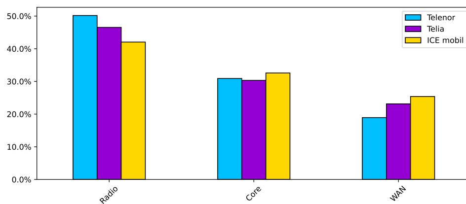
Figur 7.2: Metning i radioaksessnett, mobilkjernenettet og i nettet mellom mobilnettet og vår måletjener.
