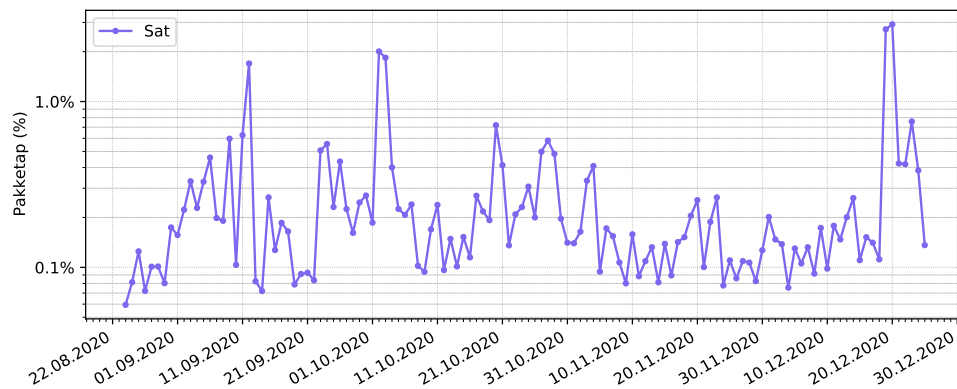
Figur 6.2: Pakketap i satellittforbindelse
